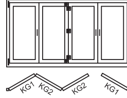
TİP 431
