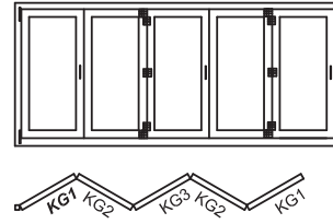
TİP 651
