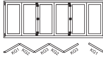
TİP 651
