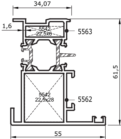
No:5562/63 Pivot Adaptörü 1,390 kg/m
