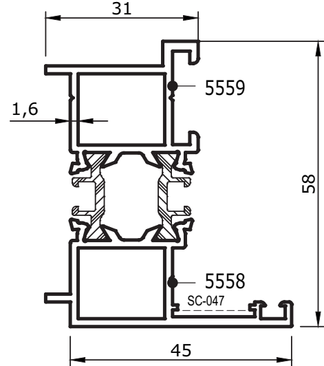
No:5558/59 Dışa Açılır Kapı Adaptörü 1.225 kg/m
