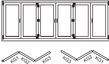
TİP 633
