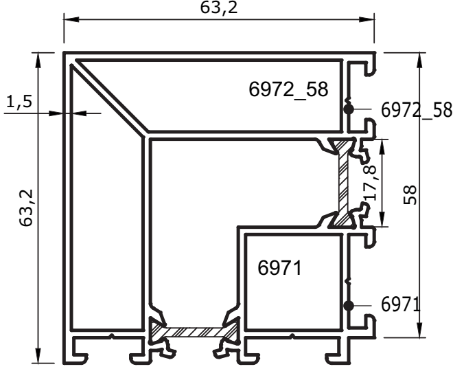
No:6971/72_58 90° Köşe Dönüş Profili 1,950 kg/m
