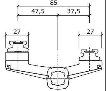
Kod : SFKM-58-079 Adaptörlü Fugalı Kapazlama Menteşe ( 10 Adet / Paket )
