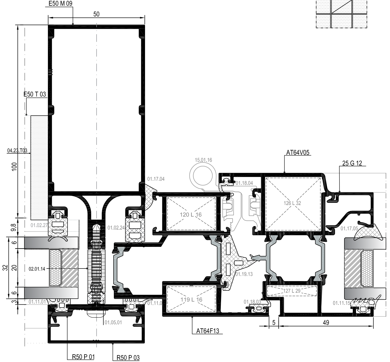
KAPAKLI CEPHE DÜŞEY DETAYI CURTAIN WALL VERTICAL DETAIL
